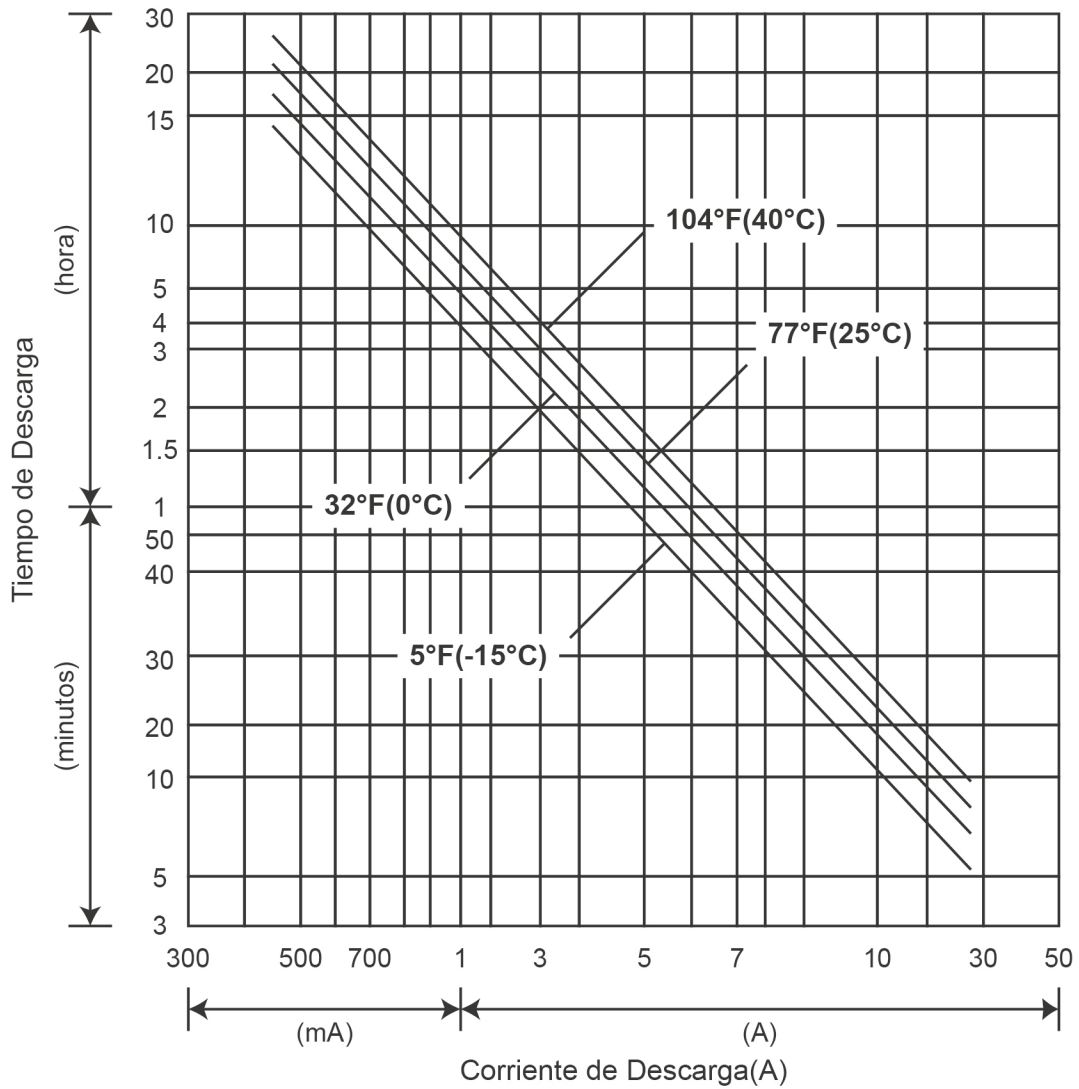
Curvas de Descarga 77°F(25°C)
