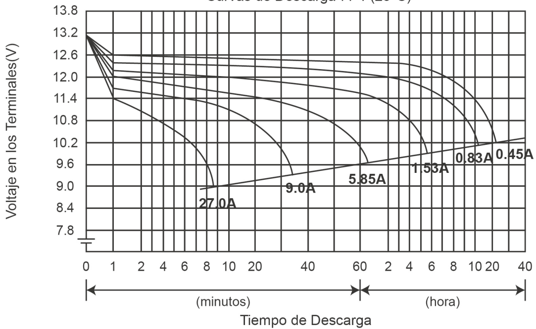
Curvas de Descarga 77°F(25°C)
